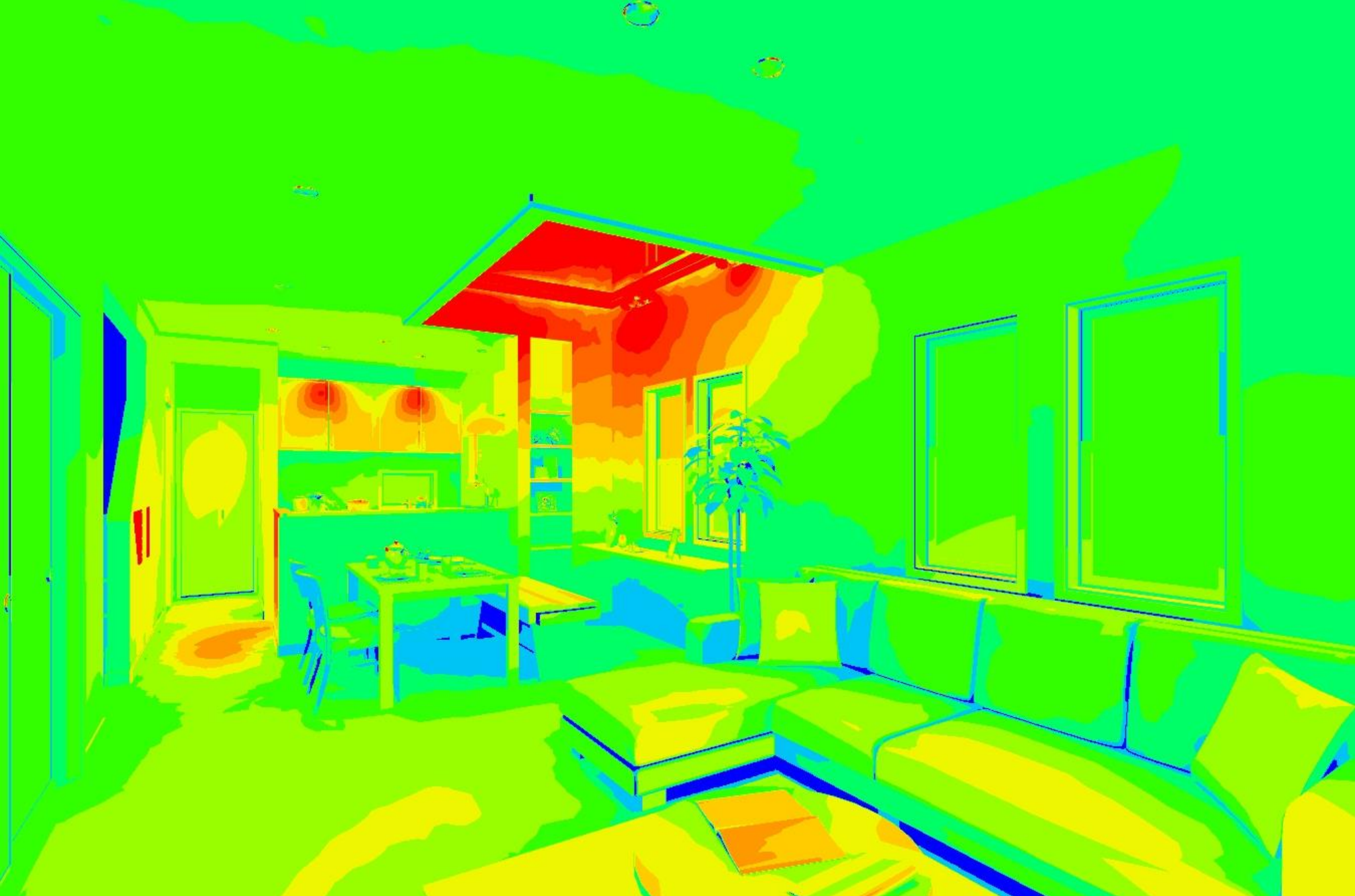
【照度分布図】 冬至 12:00
