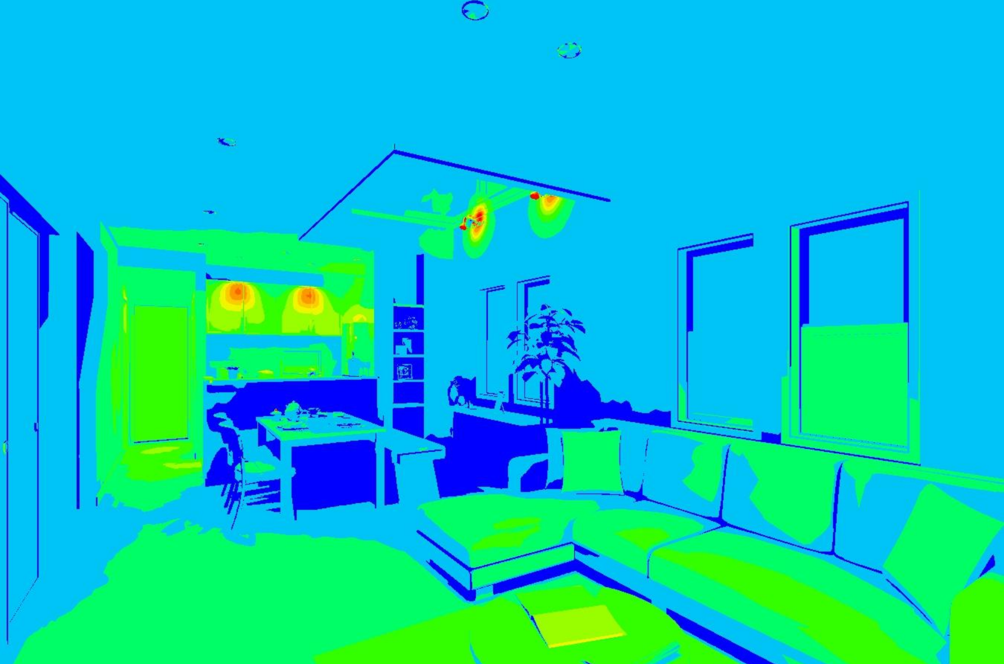
【照度分布図】冬至 8:00
