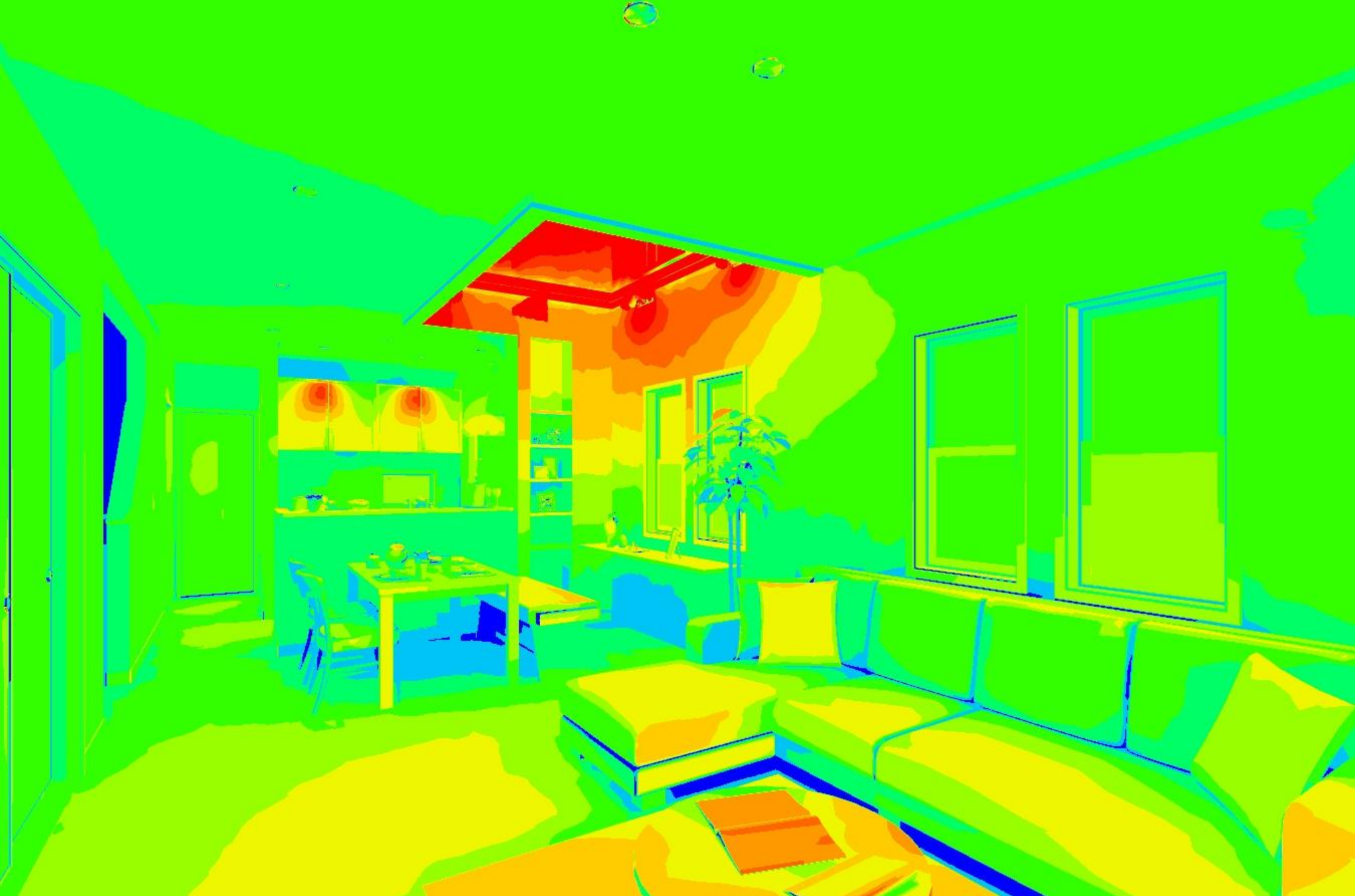
【照度分布図】冬至 13:00
