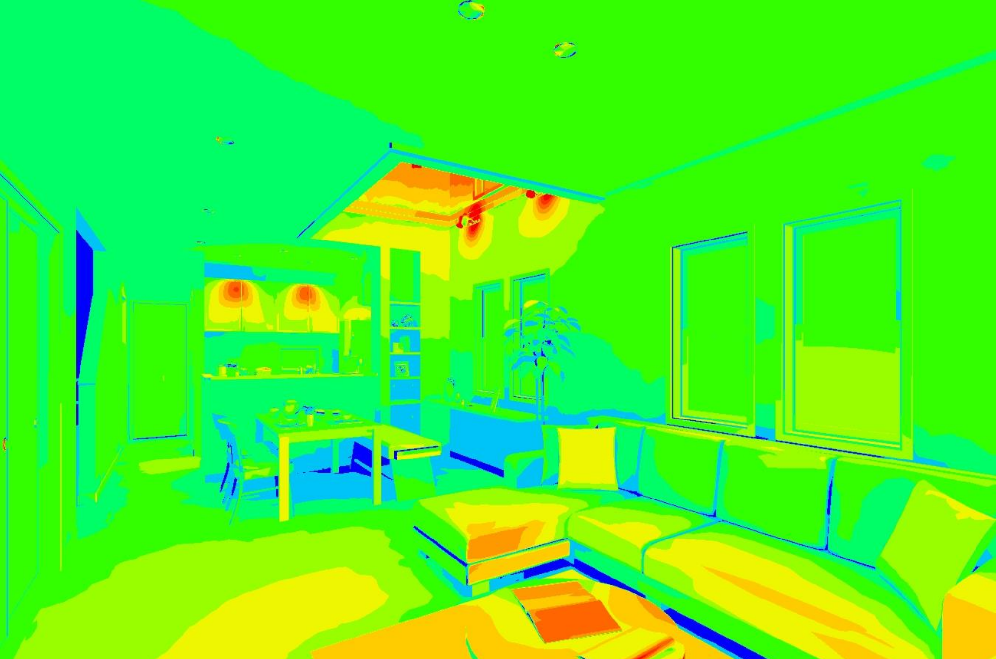
【照度分布図】冬至 14:00
