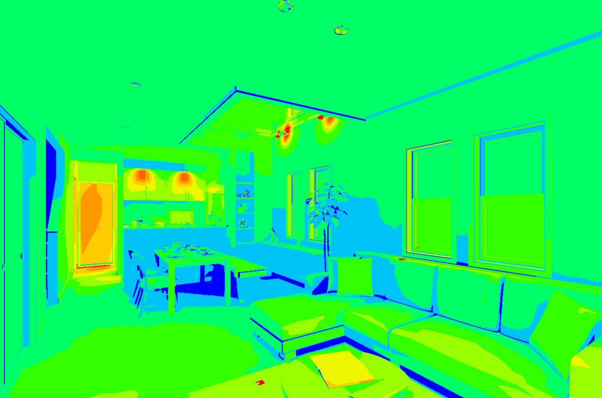
【照度分布図】冬至 10:00
