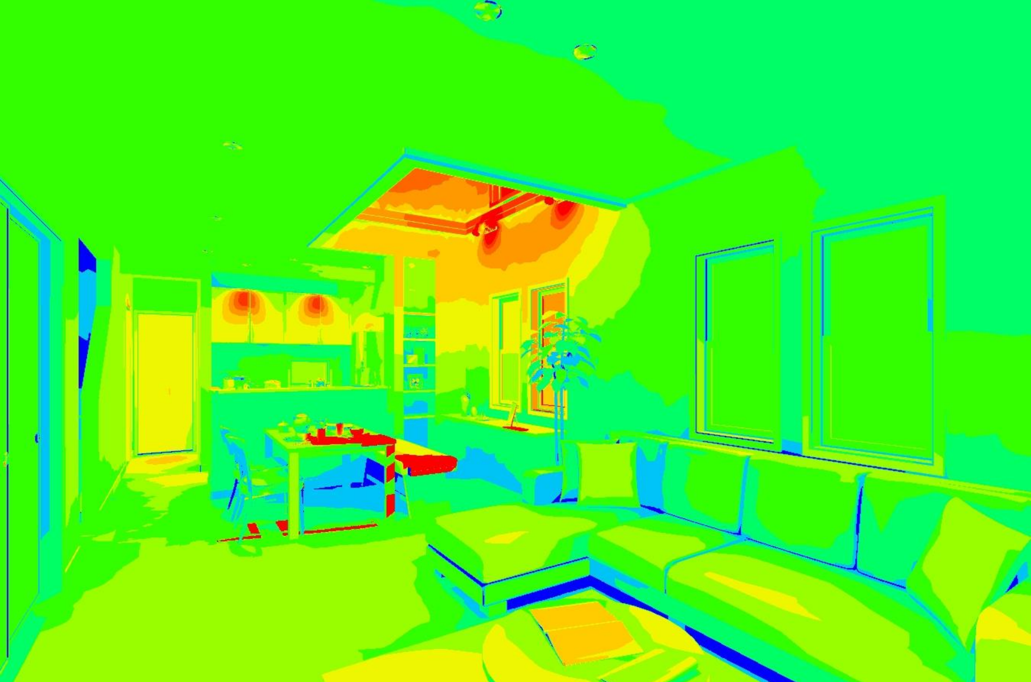
【照度分布図】冬至 11:00
