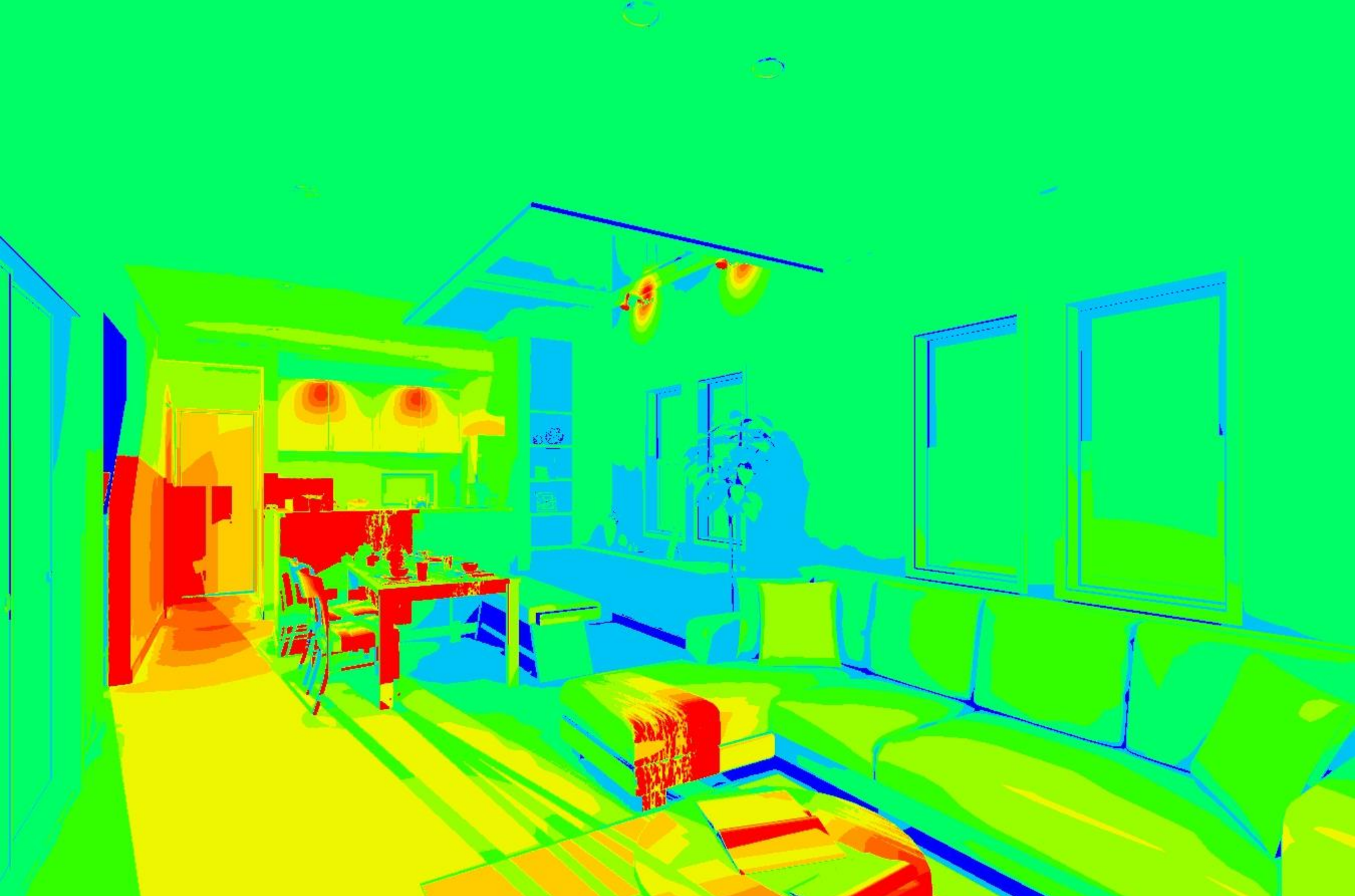
【照度分布図】冬至 16:00
