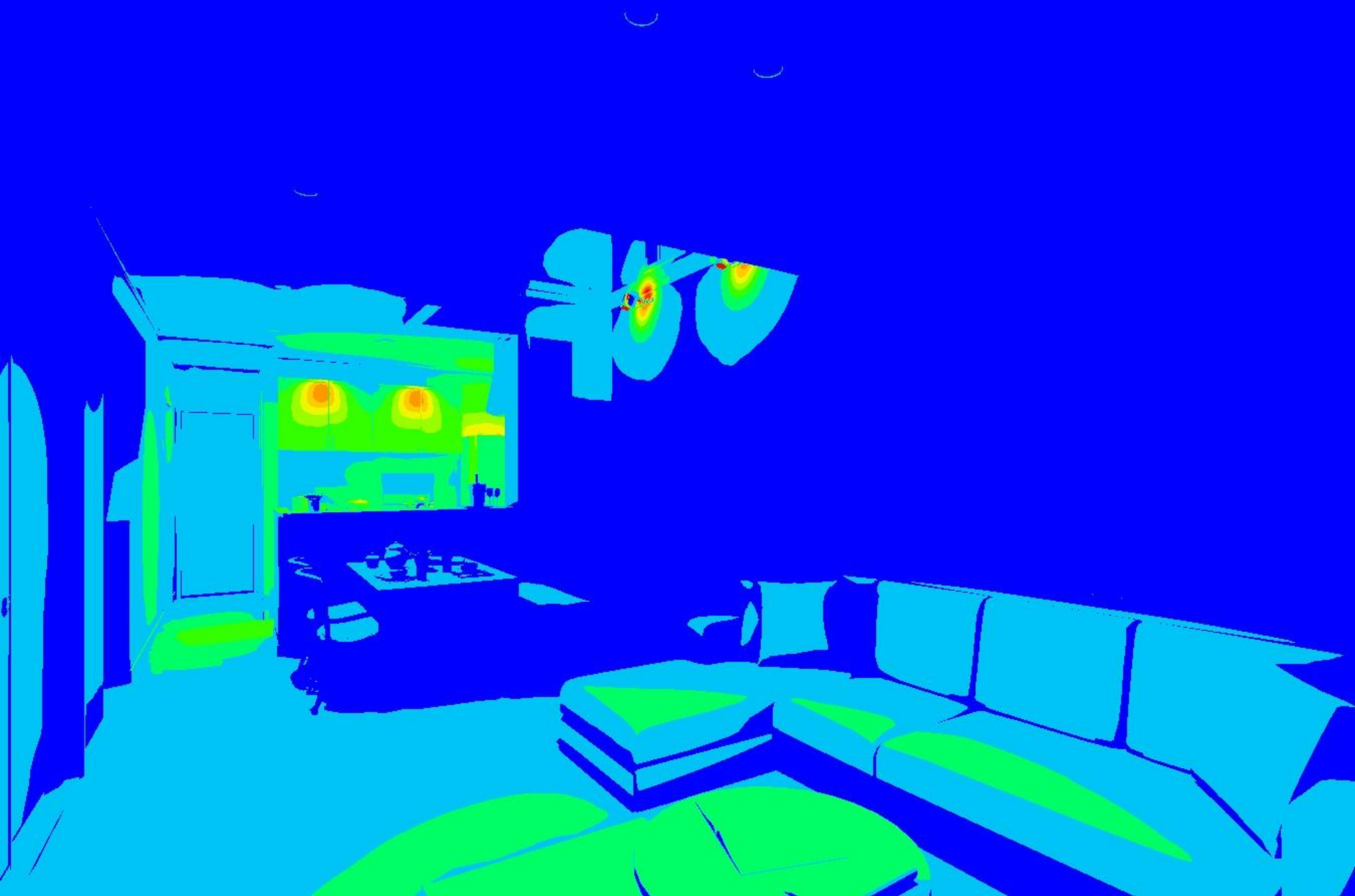
【照度分布図】冬至 17:00
