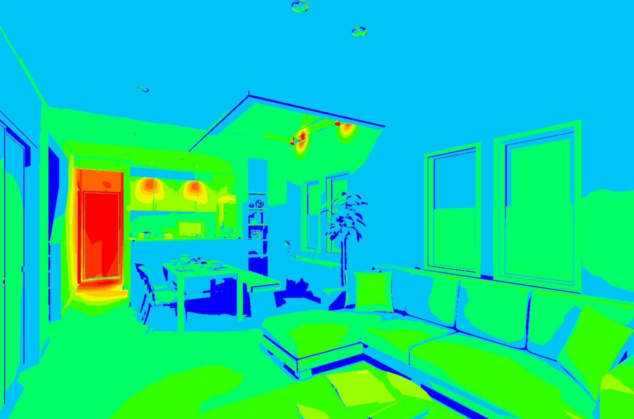
【照度分布図】冬至 9:00
